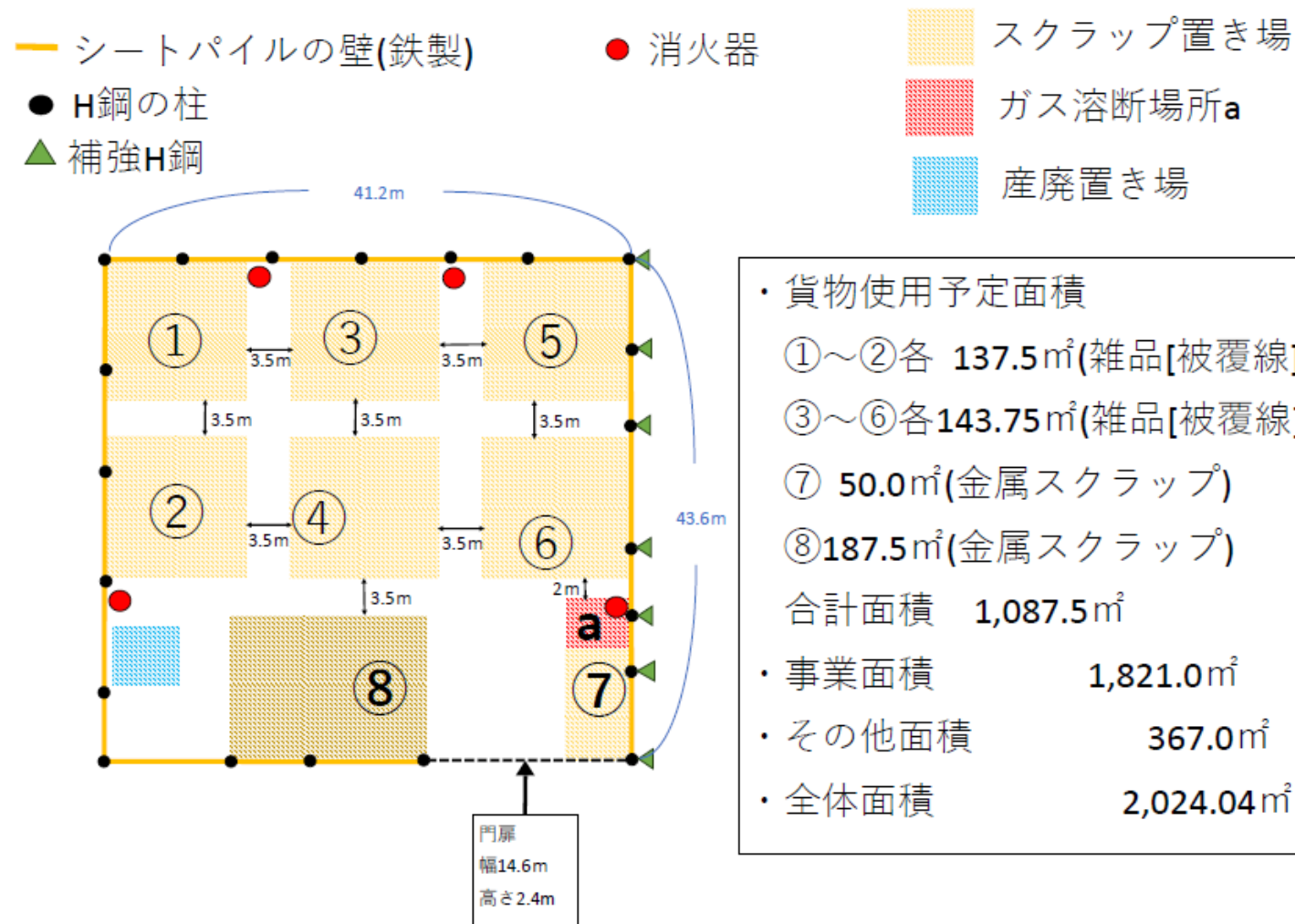
夏見工場第5ヤード 平面図
